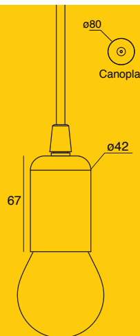
PD 1600 - 1 X E27
