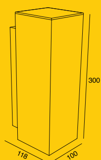
AR 112/2 - 2X E27 PAR20 OU BULBO
