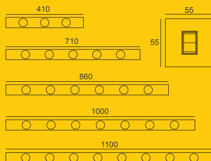
AR 163 - 3X E27 40W
